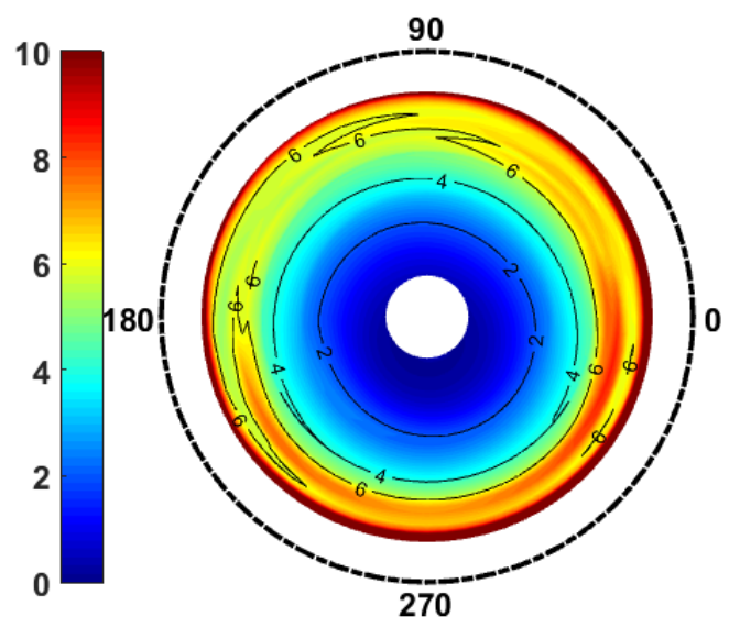
(d) Elemental Profile Drag (lbs/ft), R_{span} = 22.8 ft
